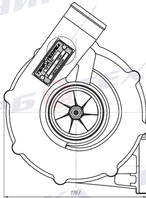
Рис.2 Остальное см. рис.1 ТКР 70.13.13-02 (левый)
