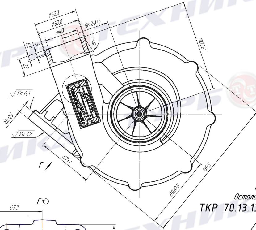
Рис.1 ТКР 70.13.13-01 (правый)
