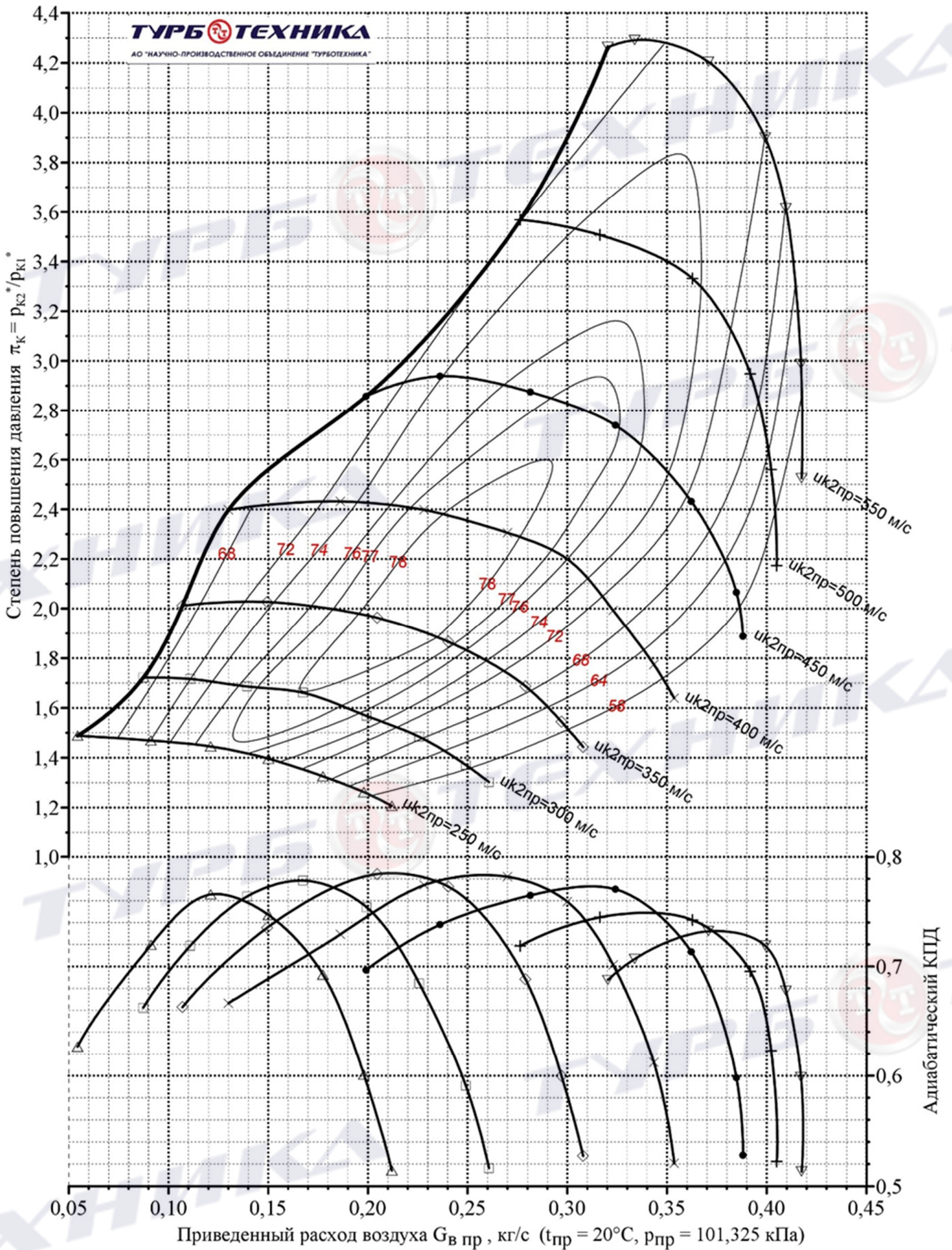
Характеристика компрессора ТКР 70.13.13
